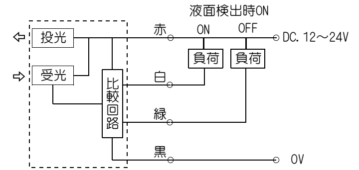
電気回路ブロック図
